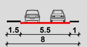
PRESJEK E-E
