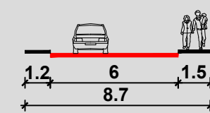
PRESJEK D-D
